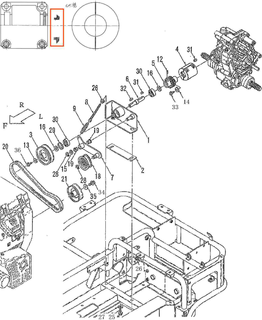
チェーンカップリング オイルシール組付け方向
